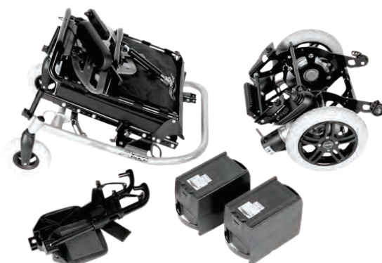
rozložený vozík A200
